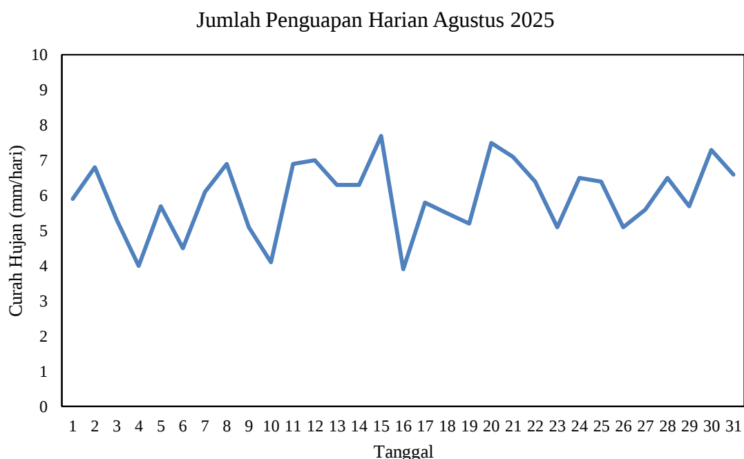
Gambar 2.8 Grafik Jumlah Penguapan Harian bulan Agustus 2025 di Stasiun Meteorologi Mali - Alor
