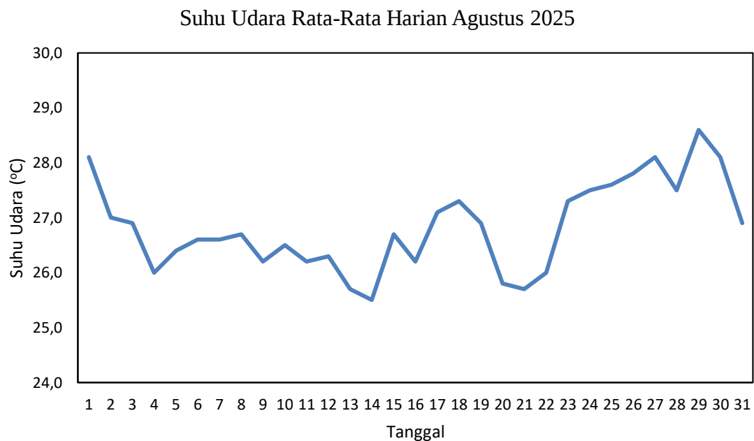
Gambar 2.1 Grafik Suhu Udara Rata-rata Harian Bulan Agustus 2025 di Stasiun Meteorologi Mali - Alor
