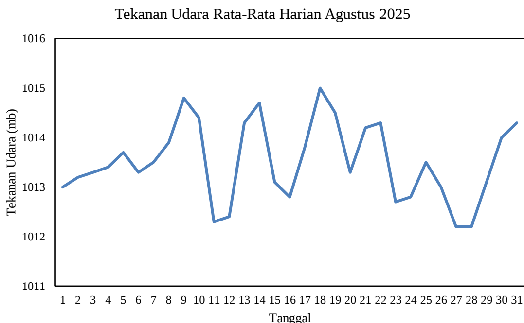
Gambar 2.6 Grafik Tekanan Udara Rata-rata Harian bulan Agustus 2025 di Stasiun Meteorologi Mali - Alor
