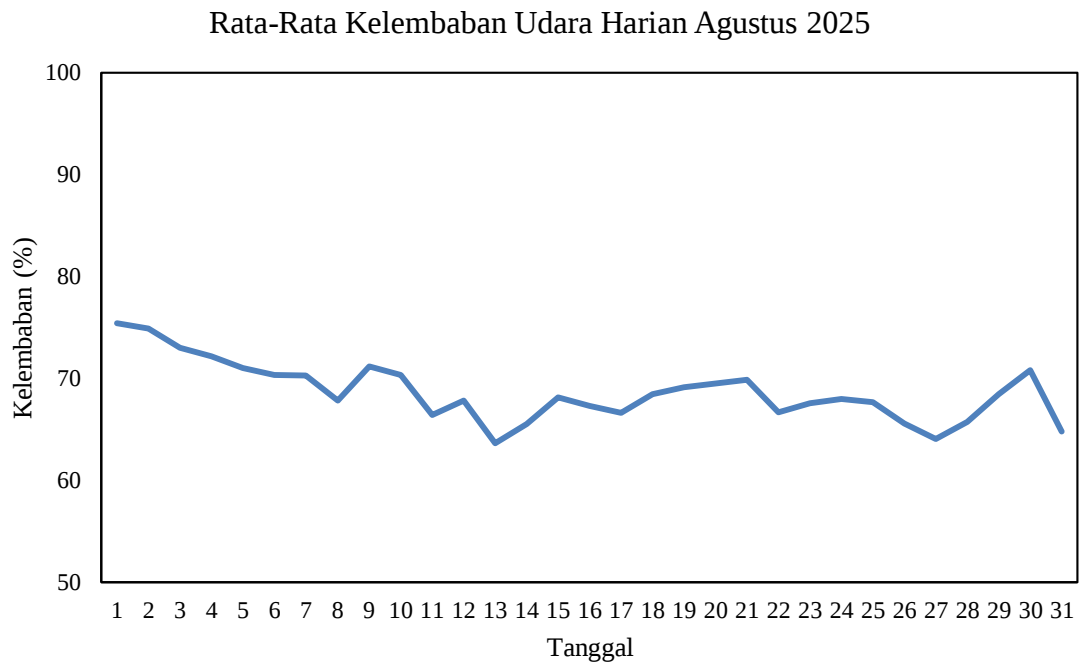
Gambar 2.5 Grafik Rata-rata Kelembaban Udara Harian Agustus 2025 di Stasiun Meteorologi Mali - Alor
