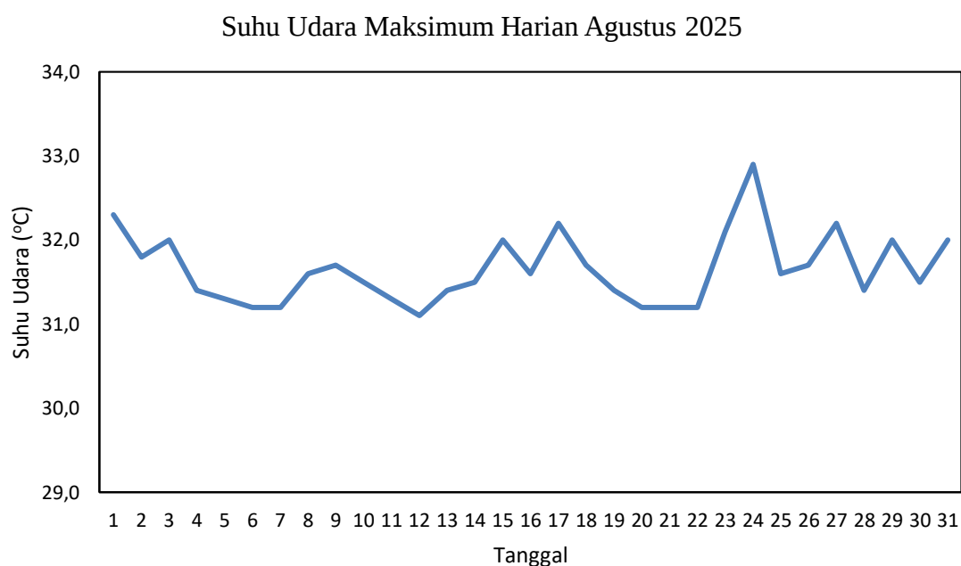
Gambar 2.2 Grafik Suhu Udara Maksimum Agustus 2025 di Stasiun Meteorologi Mali - Alor
