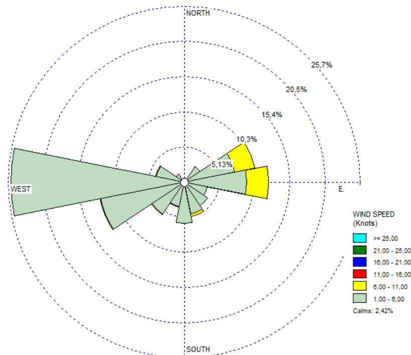
Gambar 2.9 Wind Rose Angin Permukaan Bulan Agustus 2025 di Stasiun Meteorologi Mali - Alor
