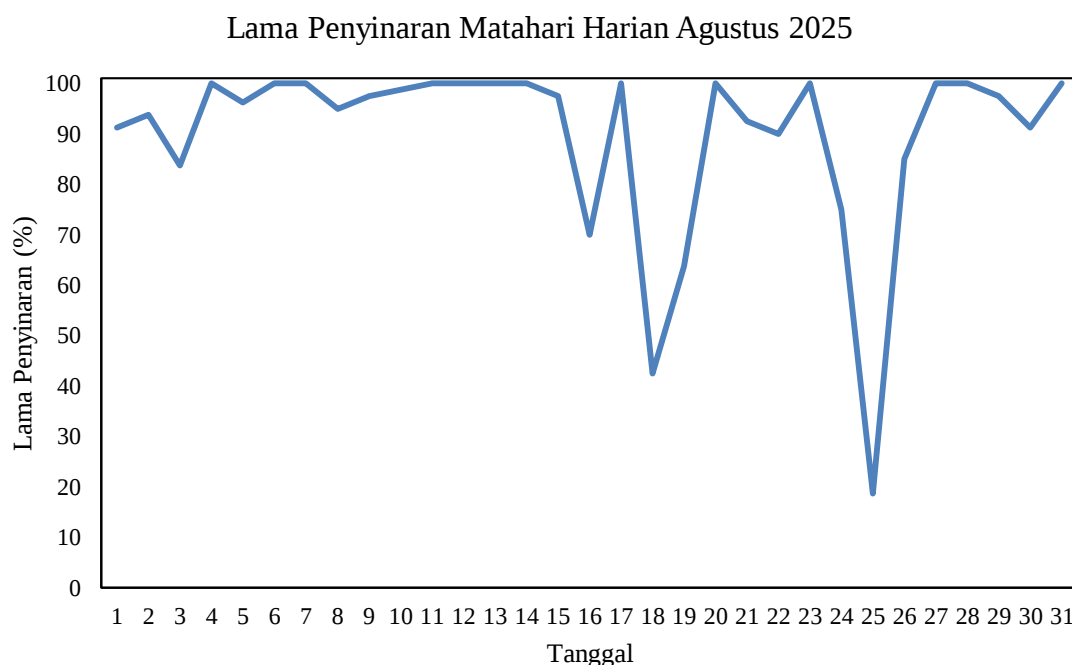
Gambar 2.7 Grafik Lama Penyinaran Matahari Harian bulan Agustus 2025 di Stasiun Meteorologi Mali - Alor
