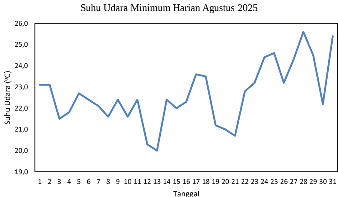
Gambar 2.3 Grafik Suhu Udara Minimum Agustus 2025 di Stasiun Meteorologi Mali - Alor
