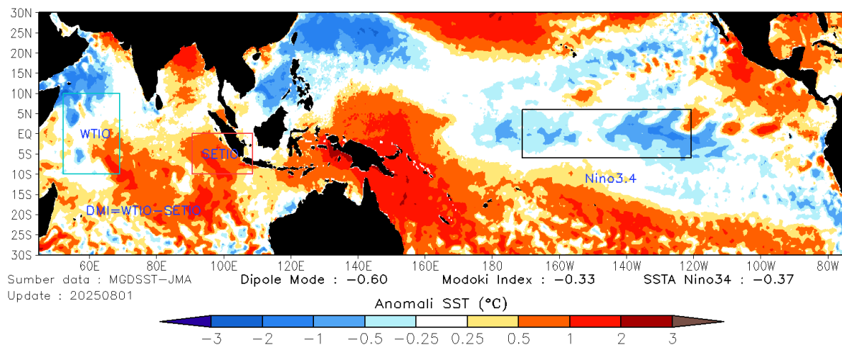
Gambar 3.2 Anomali Suhu Muka Laut di sekitar wilayah Indonesia pada Dasarian V bulan Agustus 2025
