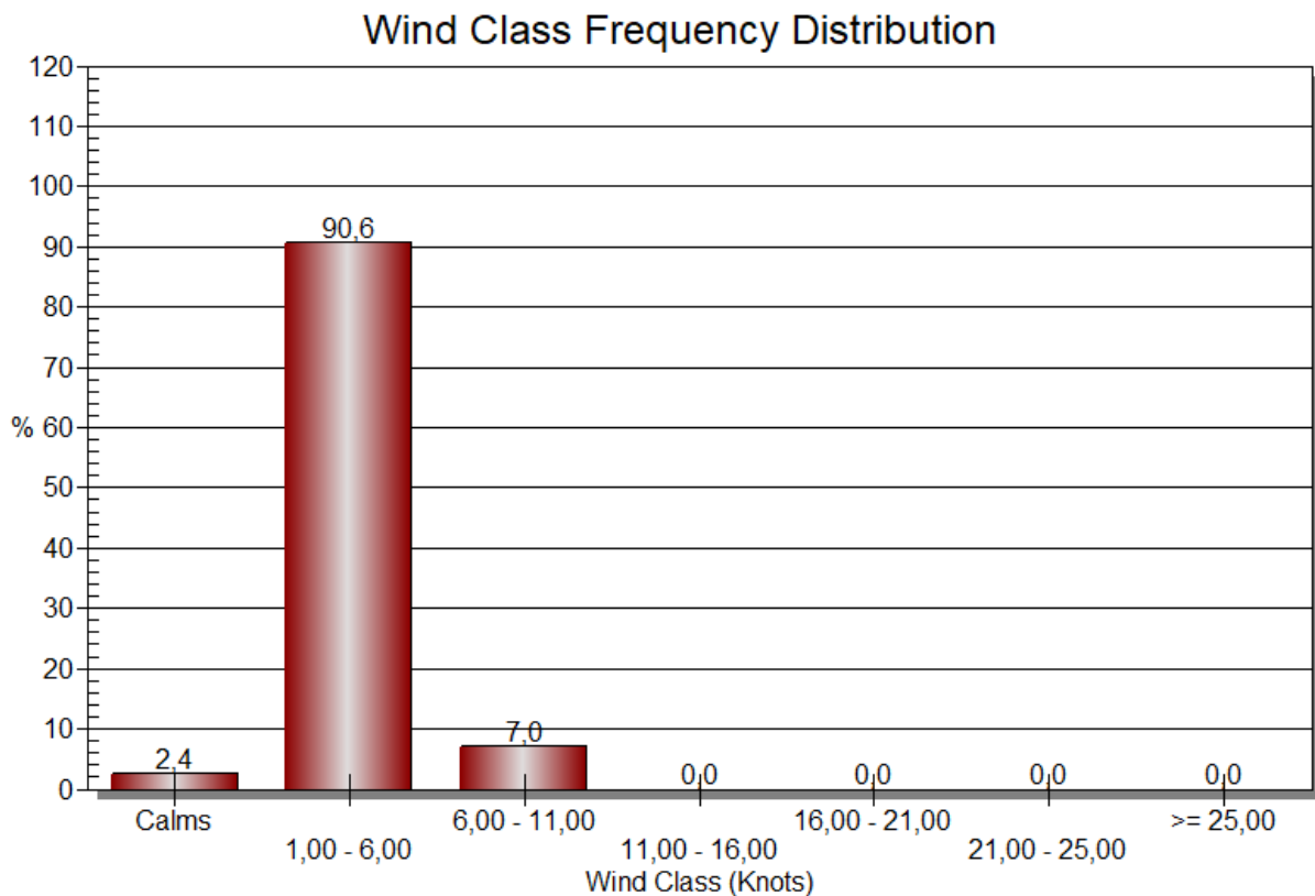
Gambar 2.10 Distribusi Frekuensi Angin Permukaan Bulan Agustus 2025 di Stasiun Meteorologi Mali - Alor
