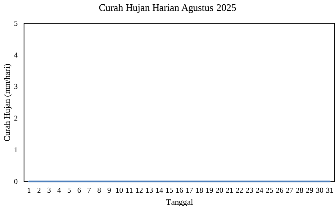
Gambar 2.4 Grafik Curah Hujan Harian Agustus 2025 di Stasiun Meteorologi Mali - Alor
